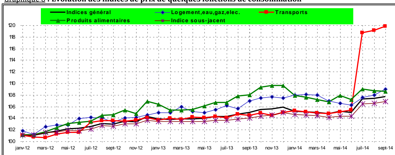
Graphique 6 : Evolution des indices de prix de quelques fonctions de consommation
